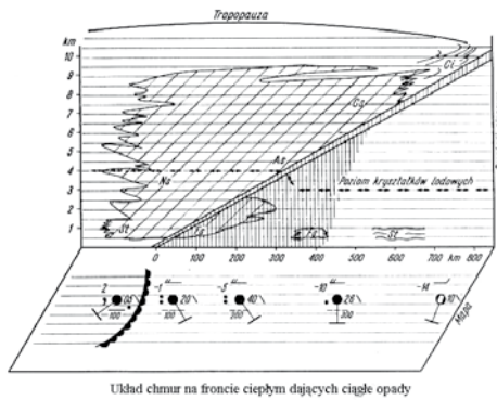
Układ chmur na froncie ciepłym dających ciągłe opady
